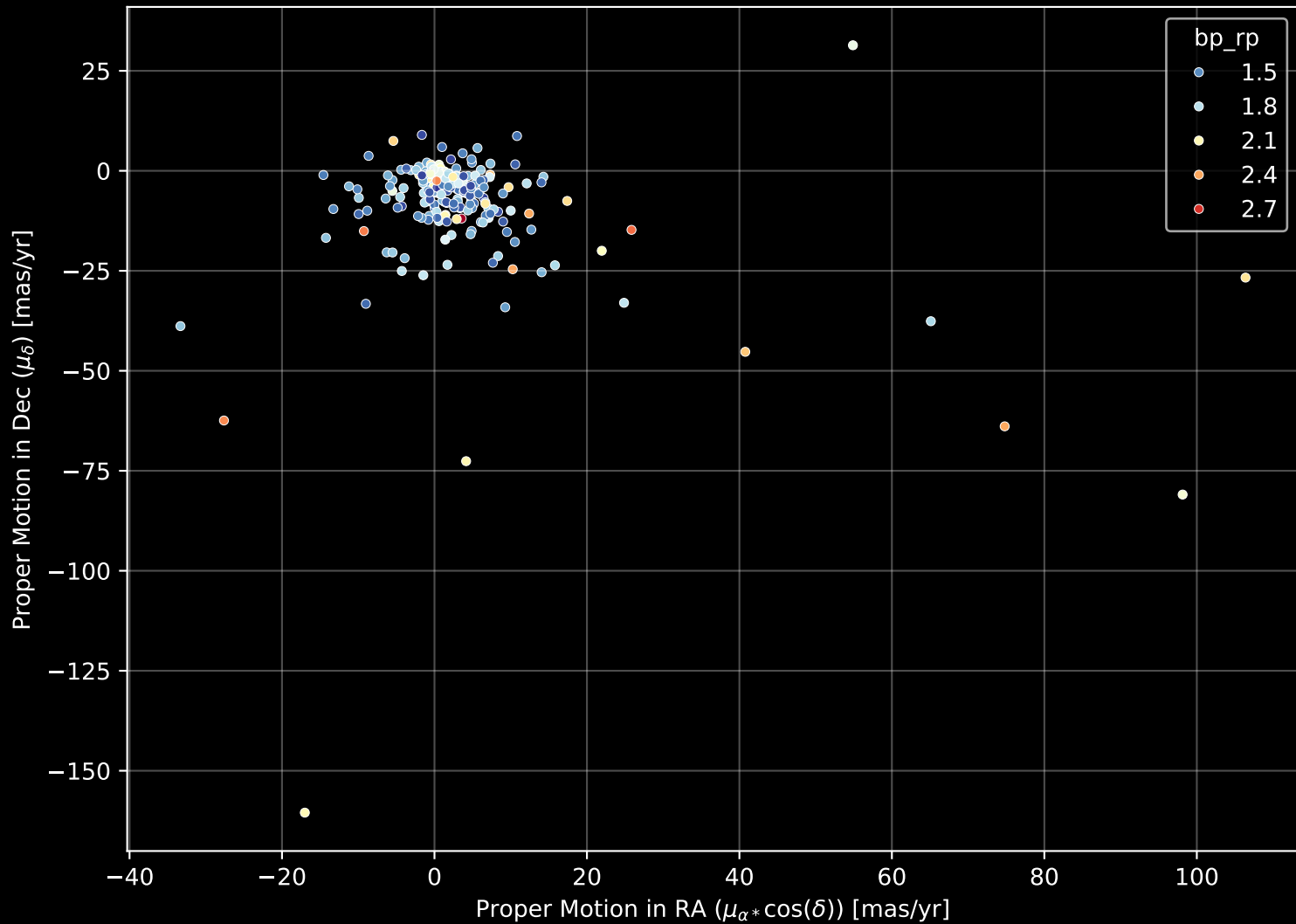
GALAH DR4 Field: [6784] Proper Motion Diagram (n= 240)
