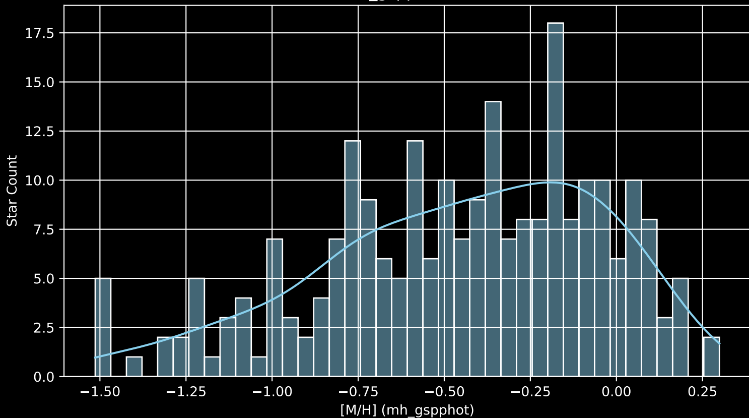
GALAH DR4 Field: [6784] [M/H] (mh_gspphot) (n= 240)
