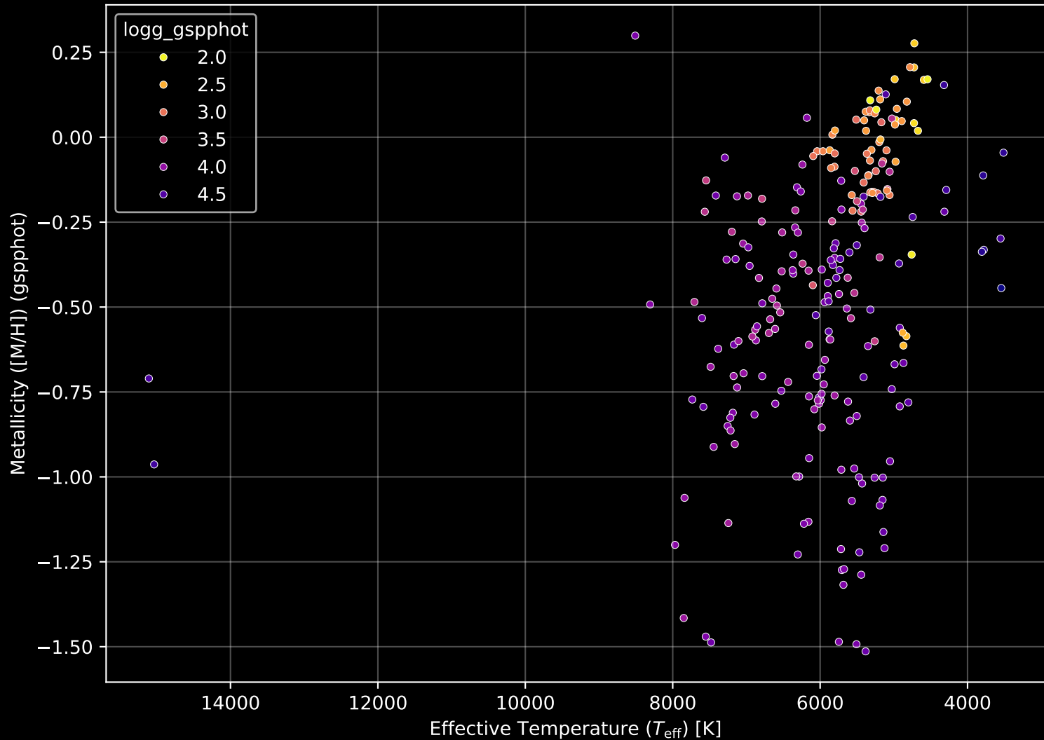
GALAH DR4 Field: [6784] Stellar Population Parameters (n= 240)
