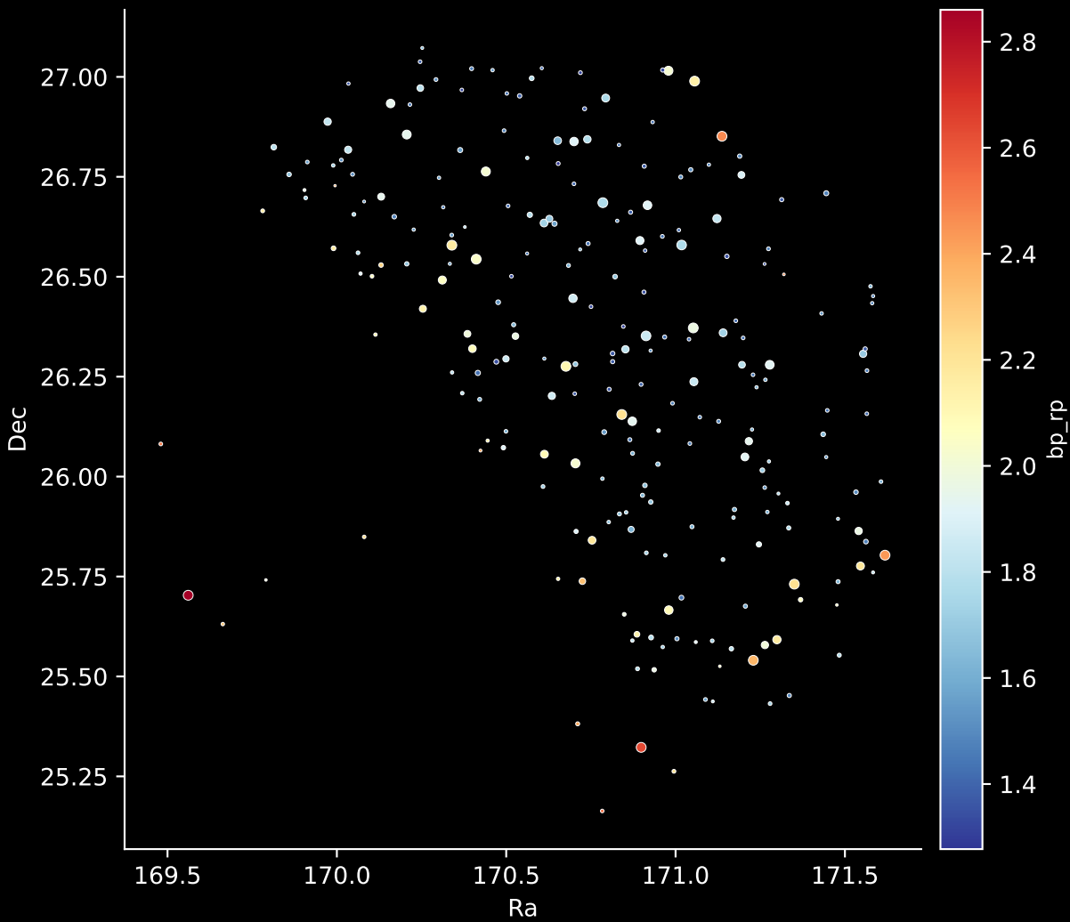
GALAH DR4 Field: [6784] Stars: 240
