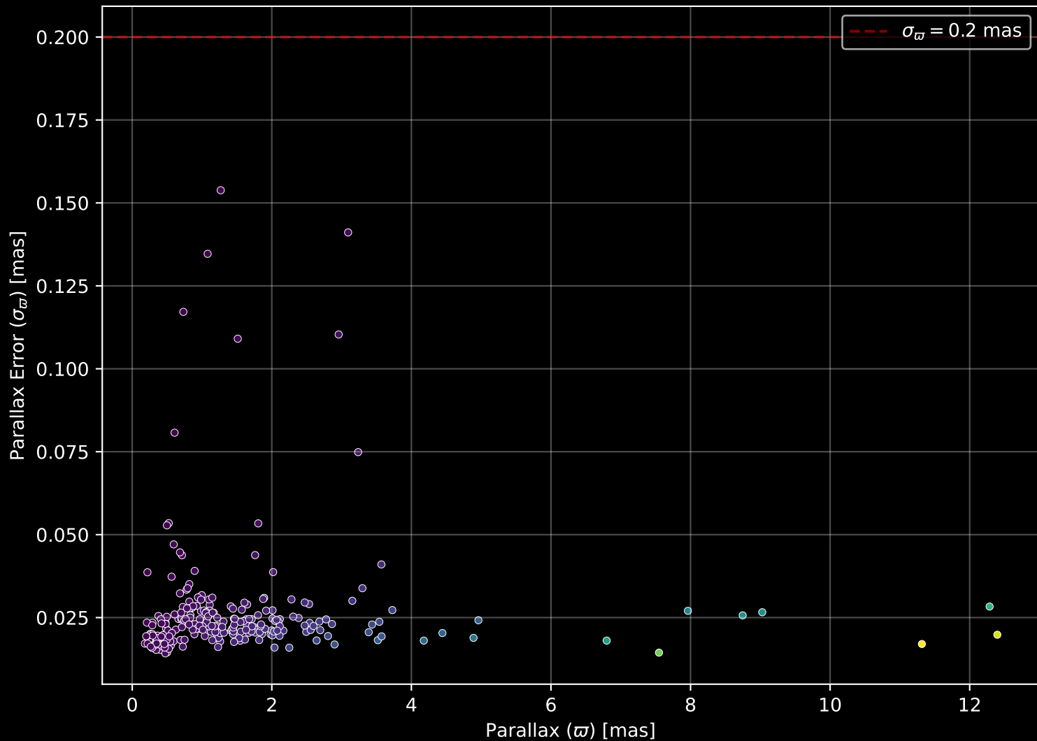
GALAH DR4 Field: [6784] Parallax Quality (n= 240)
